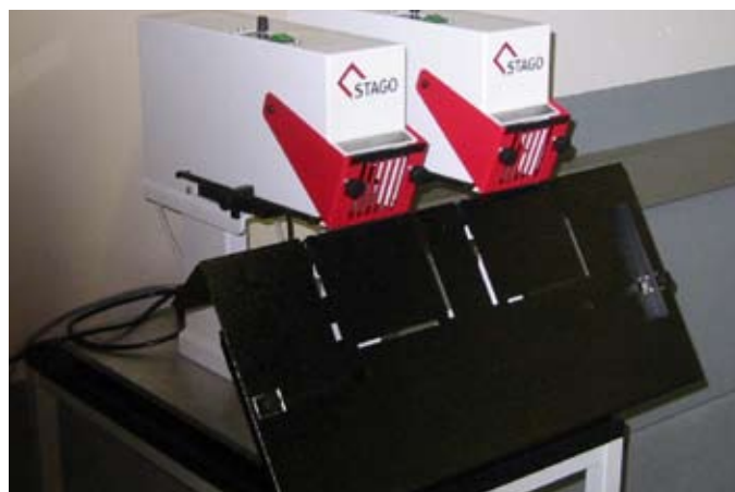
HM 6 mit 2 Heftköpfen Sonderabstand 180 mm
